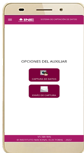
Figura 36. Menú principal.
