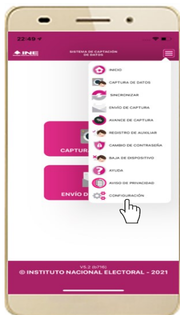
Figura 75. Configuración.
