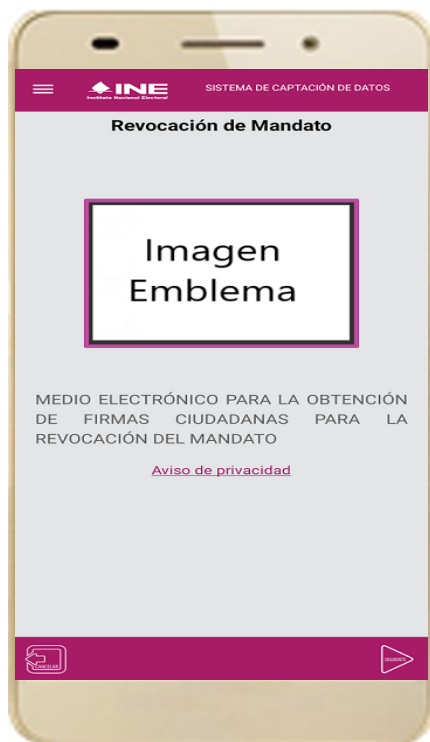
Figura 40. Descripción Proceso.
