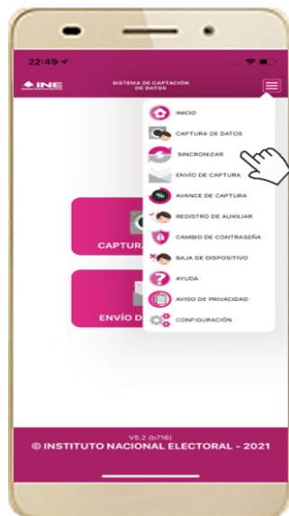
Figura 77. Sincronización Auxiliares
