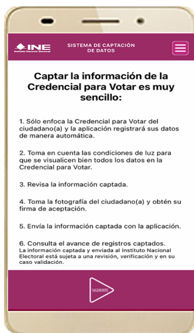
Figura 9. Instrucciones.
