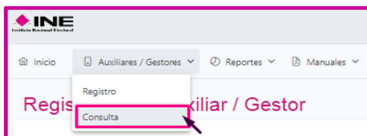
Selección “Consulta”
