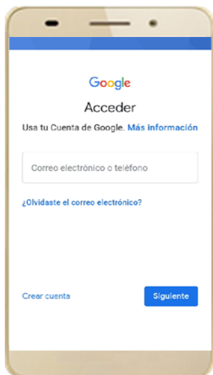
Figura 69. Autenticación Google.
