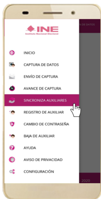
Figura 77. Sincronización Auxiliares
