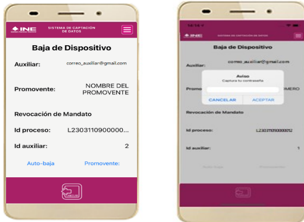
Figura 67. Contraseña Auxiliar.
