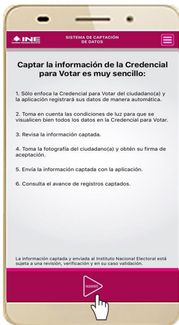
Figura 9. Instrucciones.
