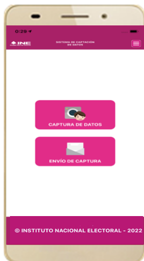
Figura 35. Menú principal.
