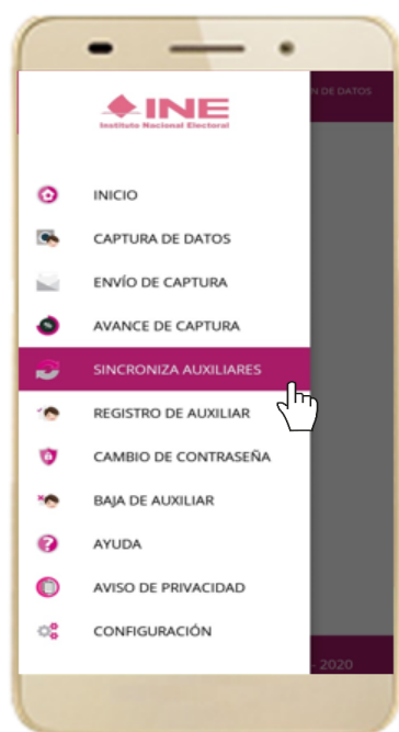
Figura 77. Sincronización Auxiliares
