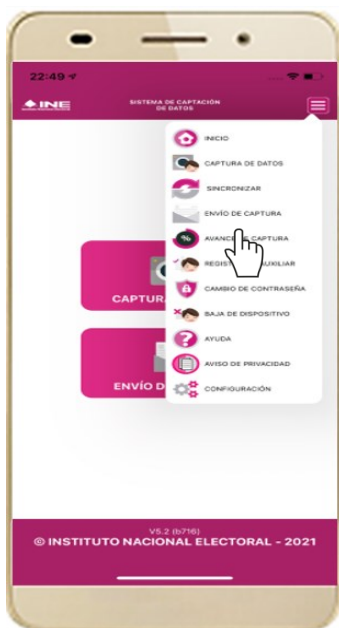
Figura 75. Configuración.
