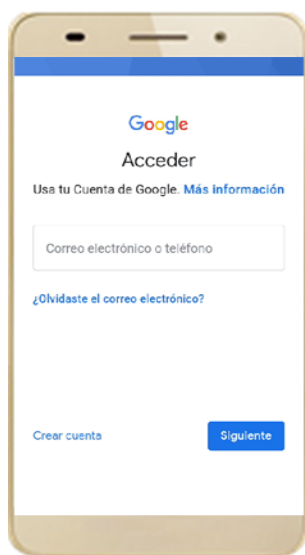
Figura 69. Autenticación Google.
