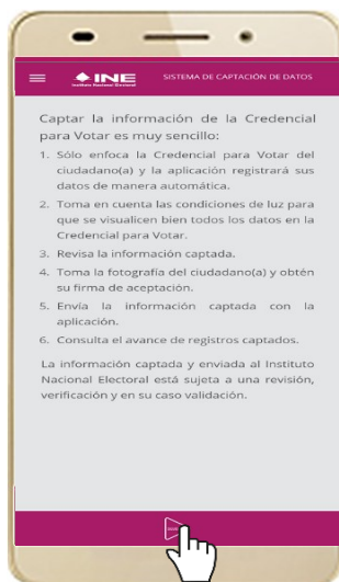
Figura 9. Instrucciones.
