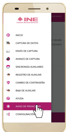
Figura 75. Configuración.
