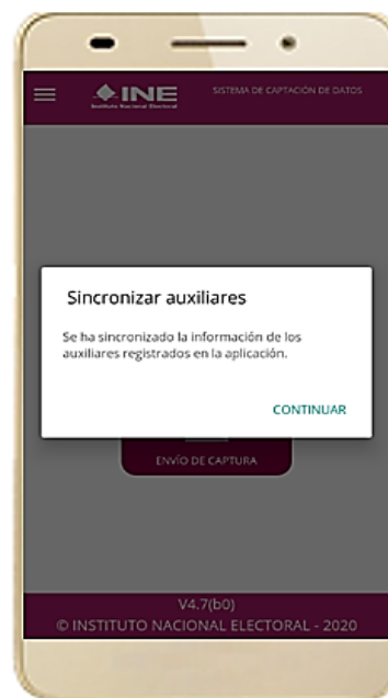
Figura 78. Mensaje Sincronización.
