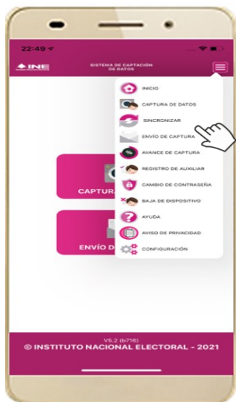
Figura 77. Sincronización Auxiliares
