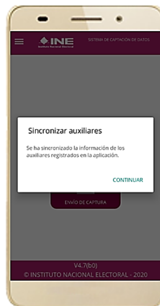
Figura 78. Mensaje Sincronización.
