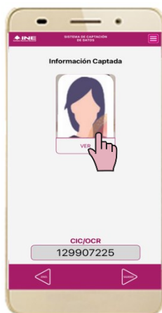
Figura 17. Información Captada
