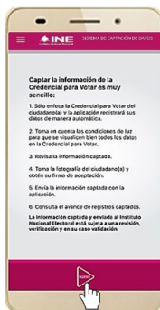
Figura 4. Instrucciones
