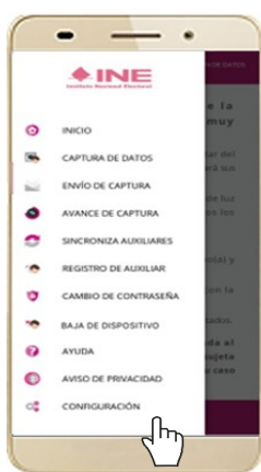
Figura 75. Configuración.
