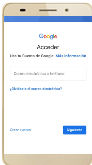
Figura 69. Autenticación Google.
