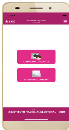
Figura 33. Menú principal.
