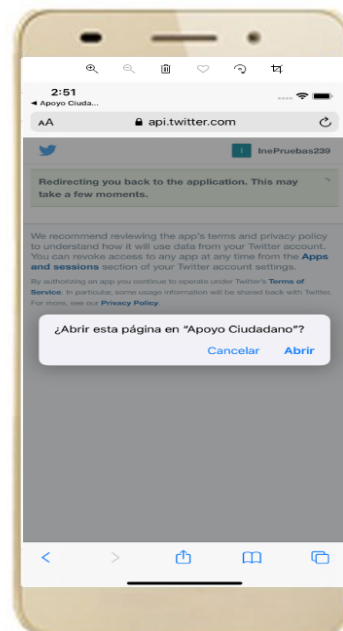
Figura 22. Autorización Twitter.
