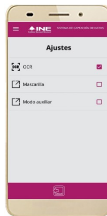
Figura 76. Configuración OCR.
