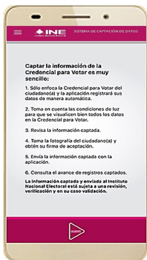
Figura 9. Instrucciones.
